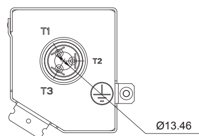
Схема подключения
